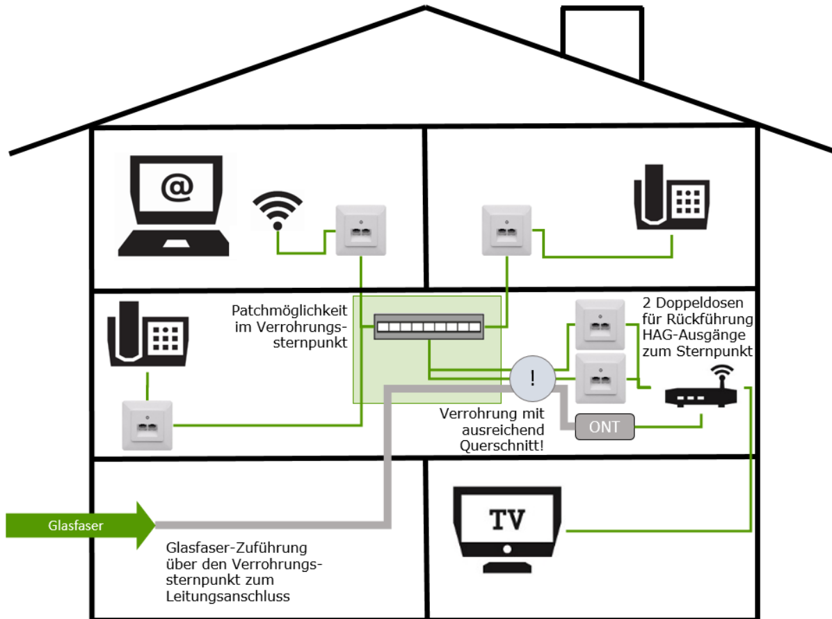
Abbildung 10: Interne Installation für Einfamilienhäuser ohne MVT
