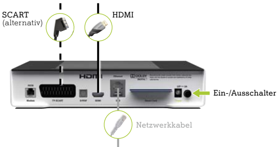
A1 Mediabox (ohne Aufnahmefunktion)
